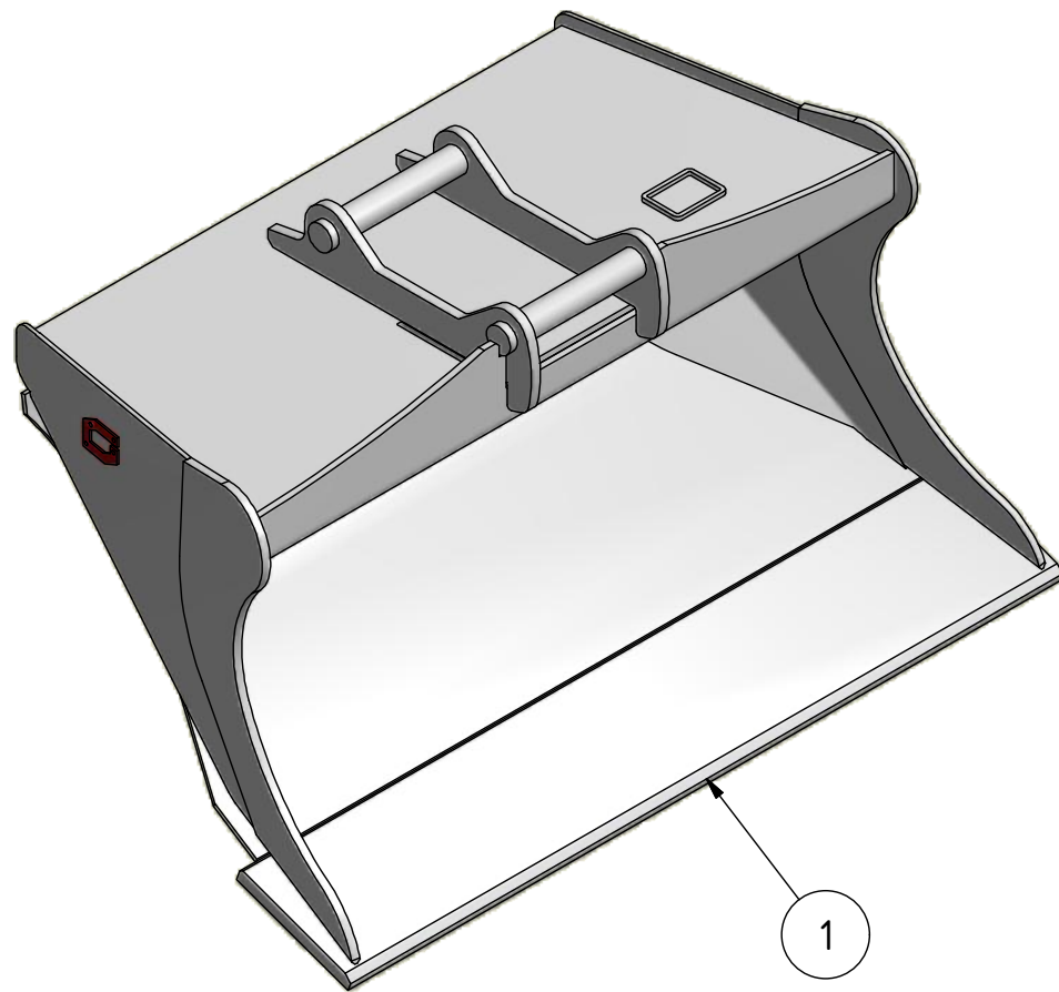
VIEW7 (1 : 10)
