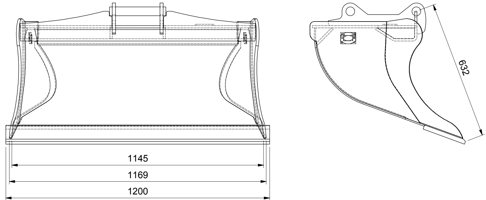
VIEW5 (1 : 10)
