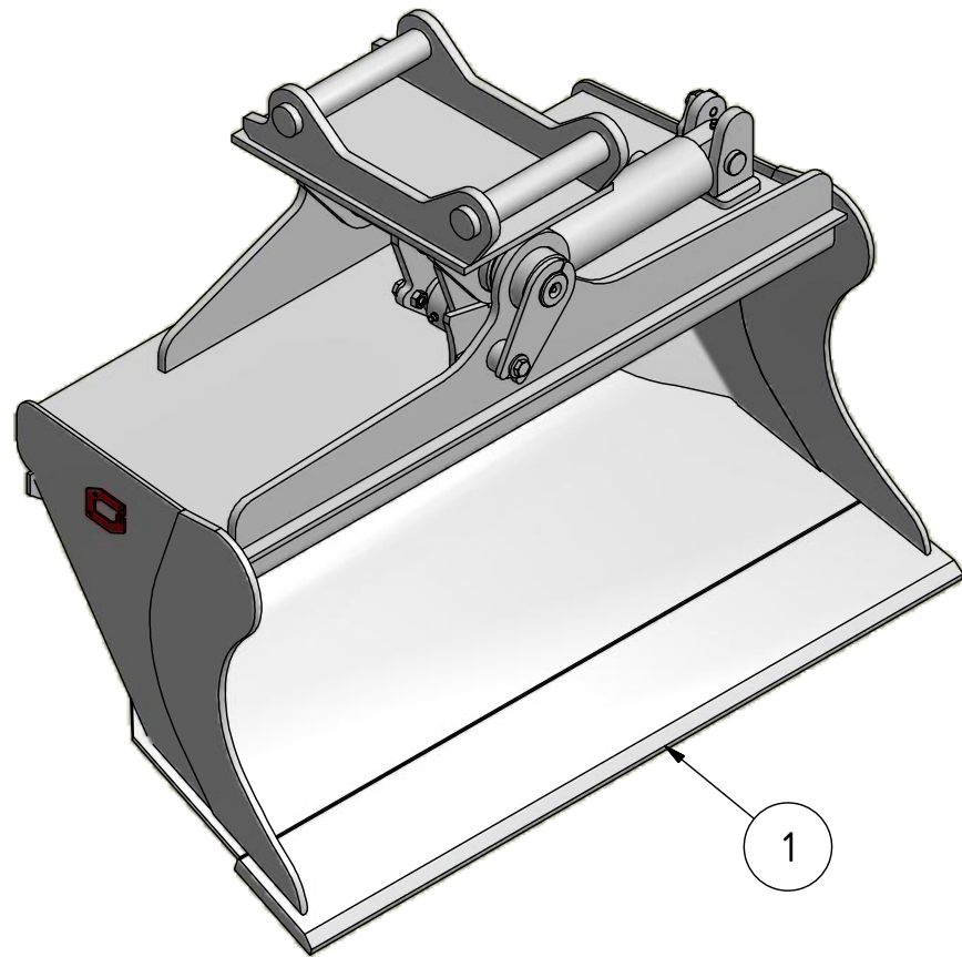
VIEW7 (1 : 10)
