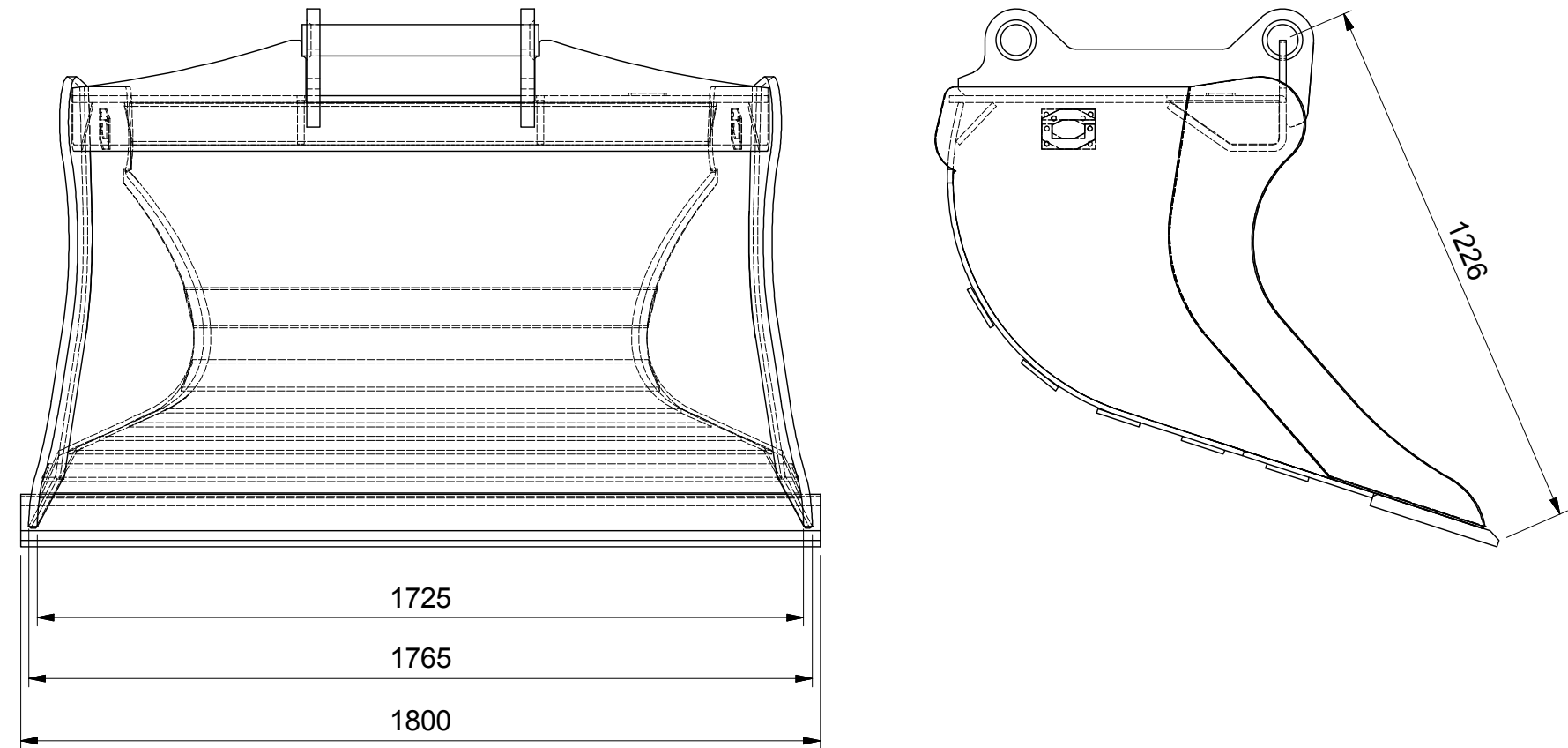
VIEW6 ( 1 : 15 )
