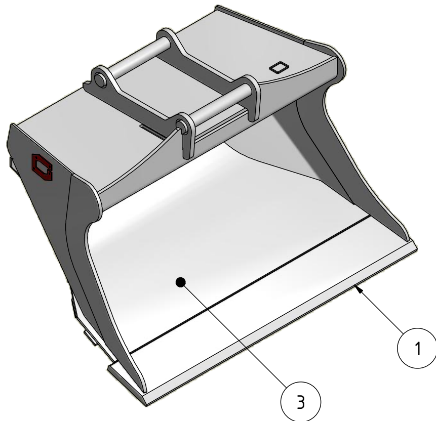
VIEW6 ( 1 : 20 )
