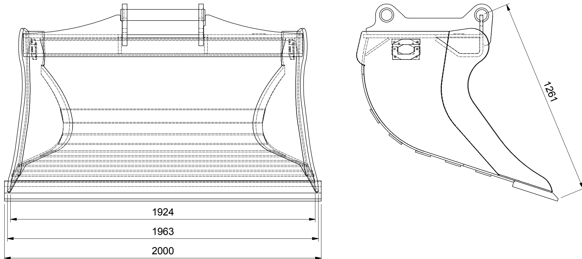
VIEW4 ( 1 : 15 )
